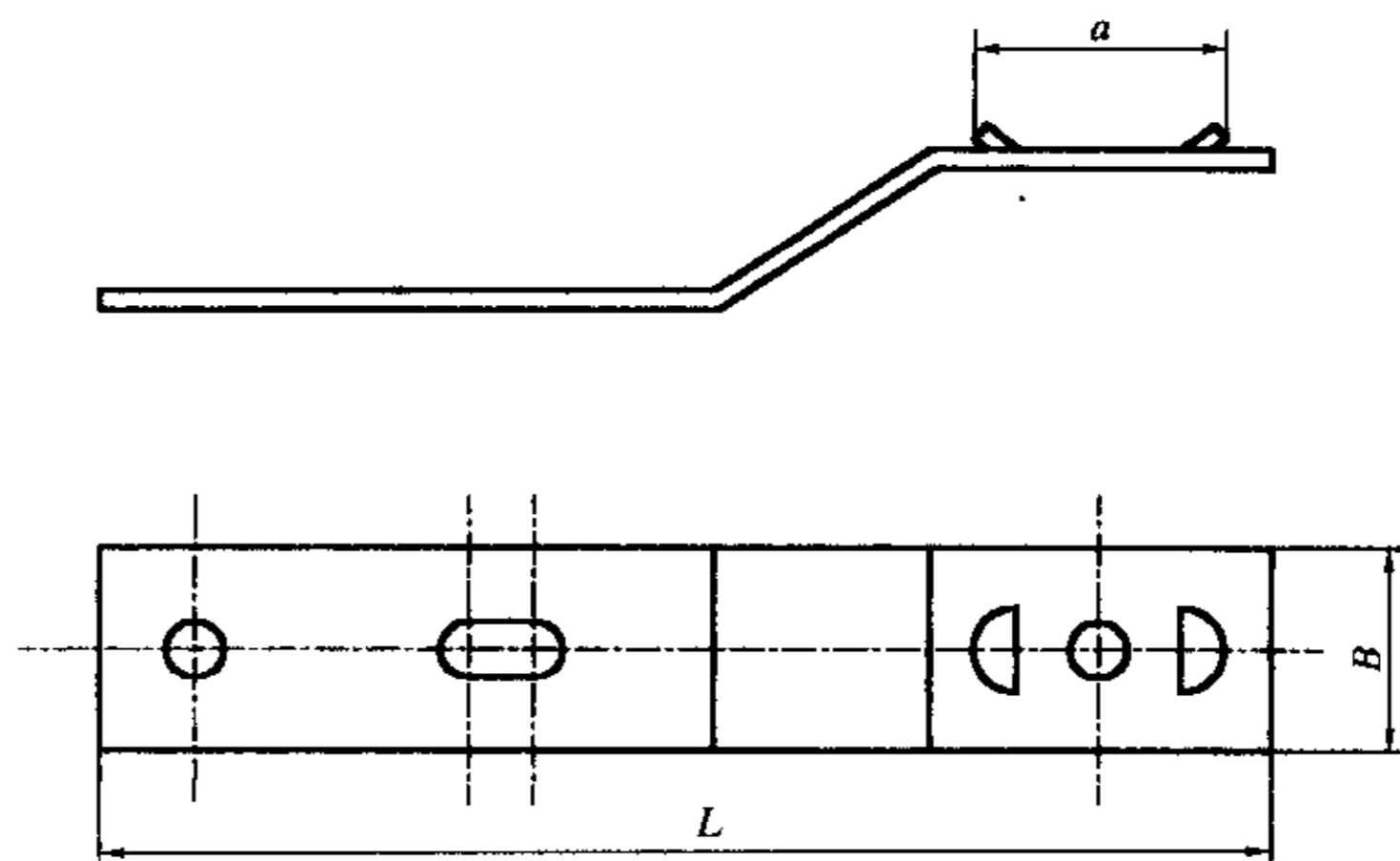
图1 单向固定片结构示意图
