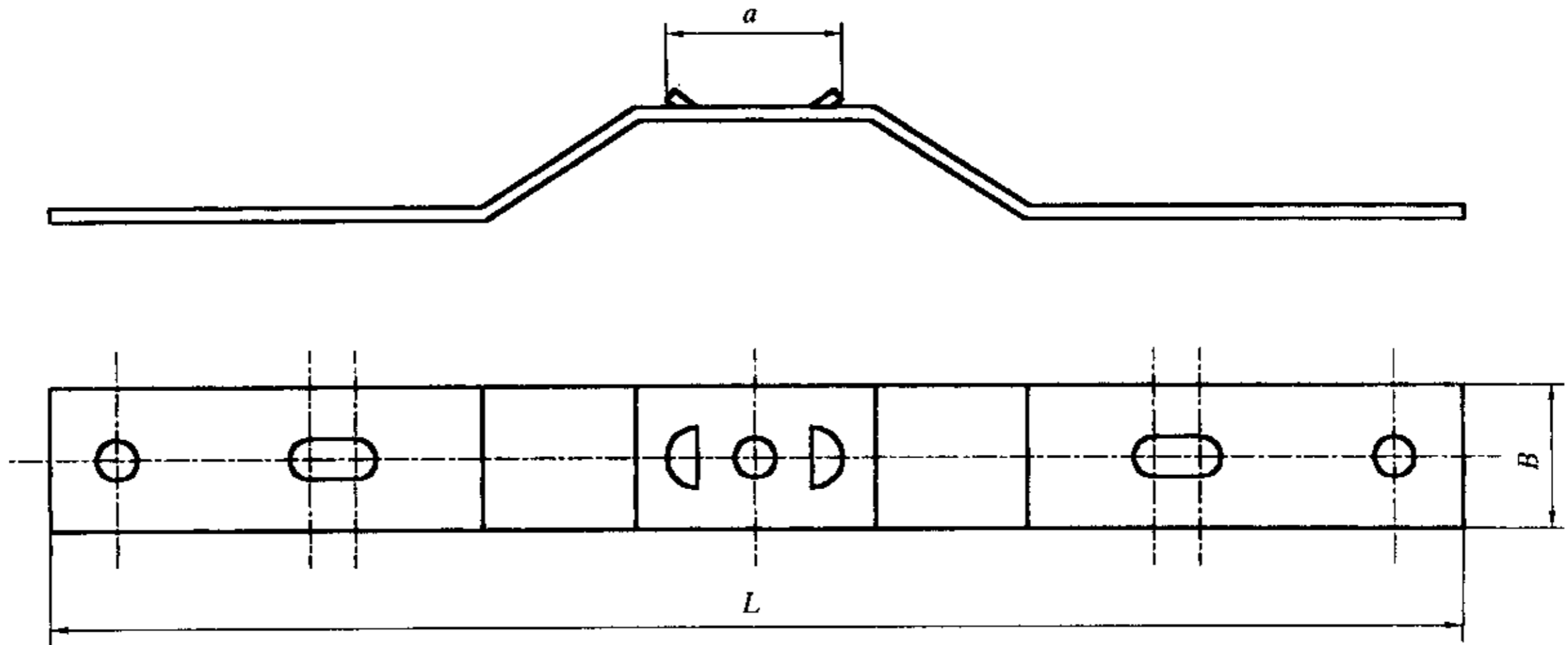
图 2 双向固定片结构示意图
